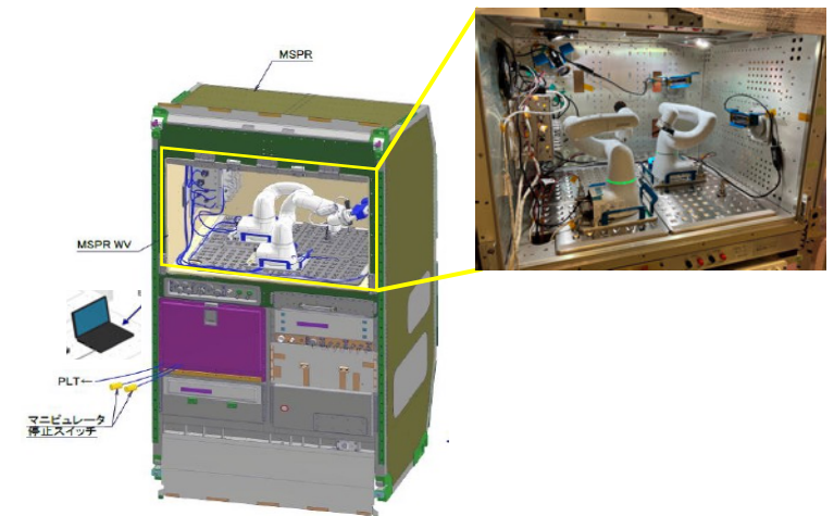
装置外観図
